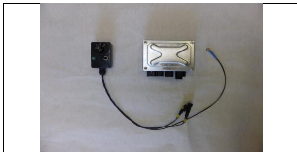
A01-14) ECU et boîtier de réglage démontés ECU and adjusting box dismantled
