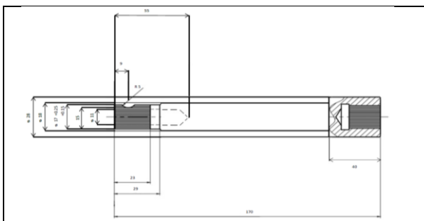
A01-15) Axe monoplace (L=170 mm) Monoplace shaft (L=170 mm)
