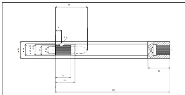
A01-16) Axe biplace (L=190 mm) Biplace shaft (L=190 mm)
